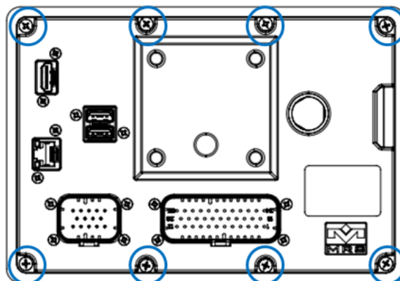
Abbildung 2: Schematische Darstellung – Rückseite des MConn 7 und Lokalisation der acht Kreuzschlitzschrauben (blaue Kreise).
